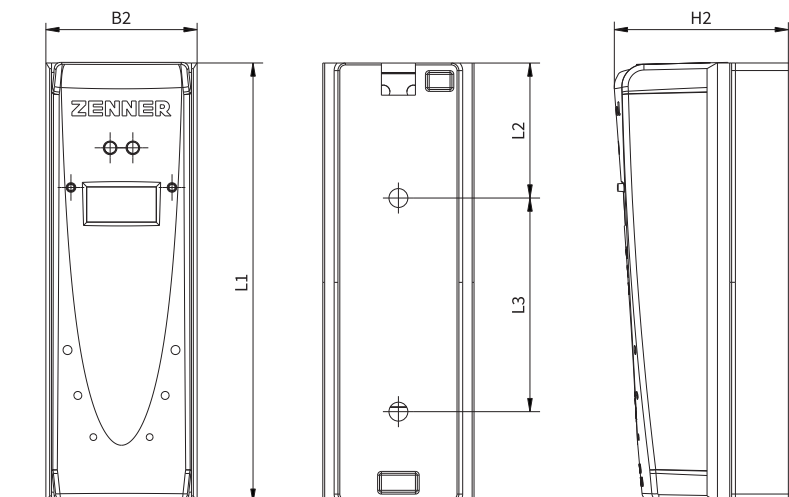
Abmessungen Splittversion
