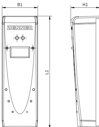
Abmessungen Kompaktversion
